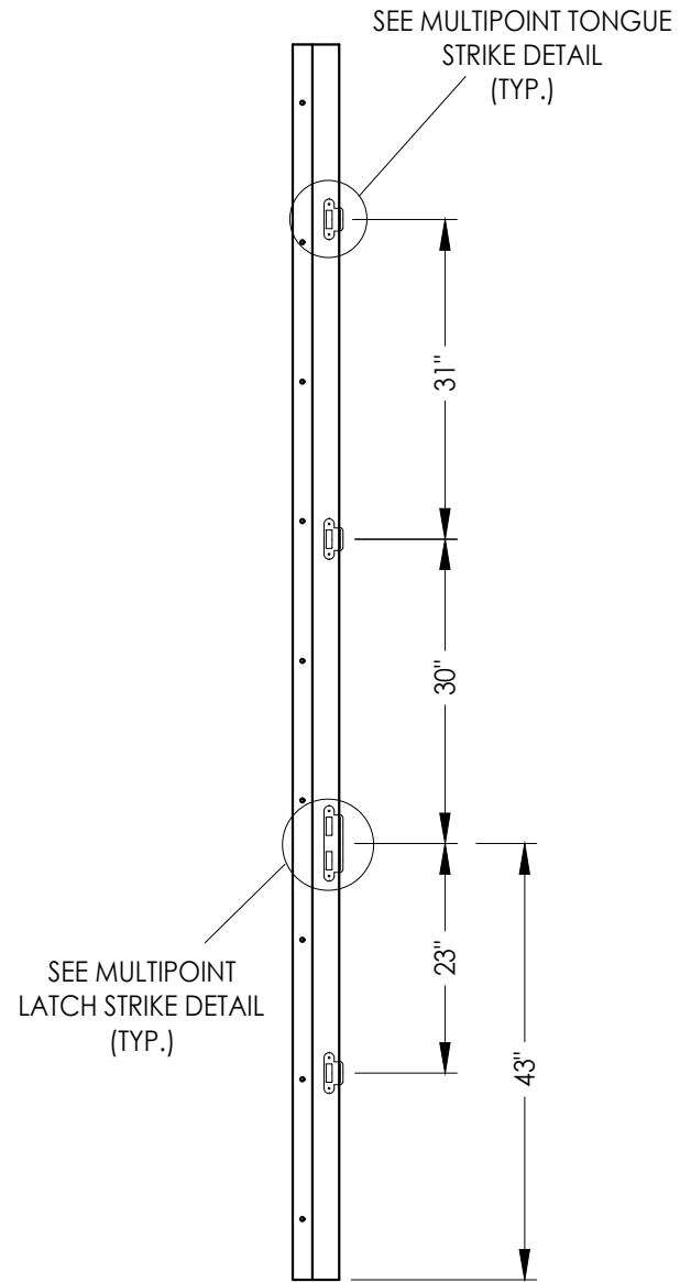
LOCK JAMB
